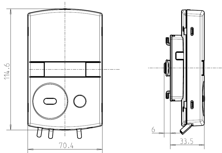
Abb. 12: Maße Rechenwerk
