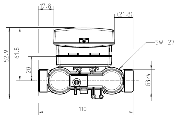
Abb. 1: Übersicht Maße Baulänge 110 mm
