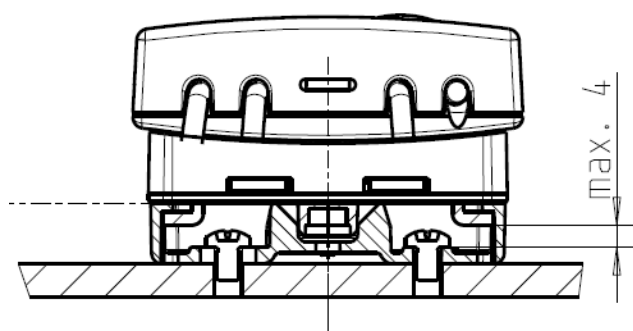
Abb. 14: Maximal zulässige Schraubenkopfhöhe (bei Verwendung der Wandhalterung)
