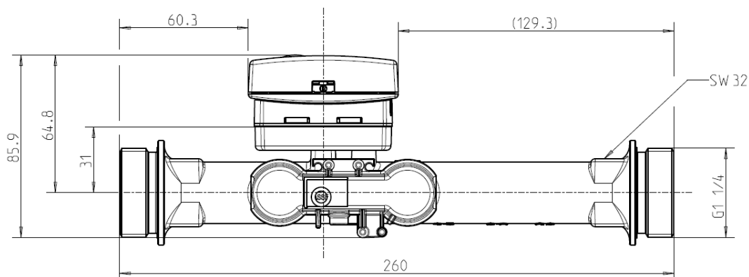
Abb. 5: Übersicht Maße Baulänge 290 mm (Gewinde)
