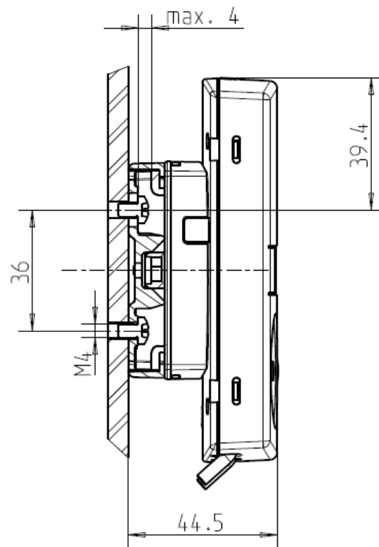
Abb. 15: Wandmontage
