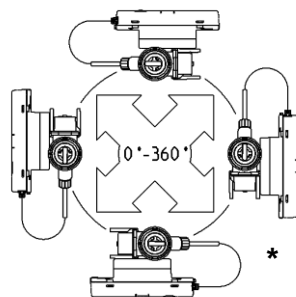
Abb. 6: Einbaupositionen
