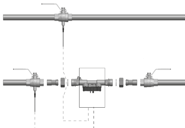
Abb. 7: Installationsbeispiel
