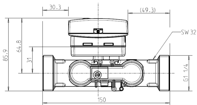
Abb. 4: Übersicht Maße Baulänge 150 mm (Gewinde)
