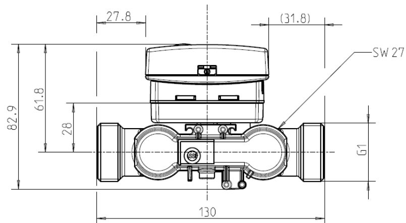
Abb. 2: Übersicht Maße Baulänge 130 mm (Gewinde)
