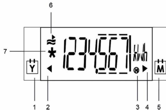
Abb. 16: LCD-Anzeige
